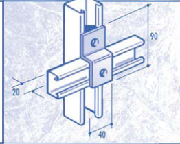
CF22 'Z' BRACKET TOP HAT
