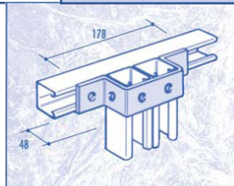
CF28 DOUBLE WIDTH TOP HAT
