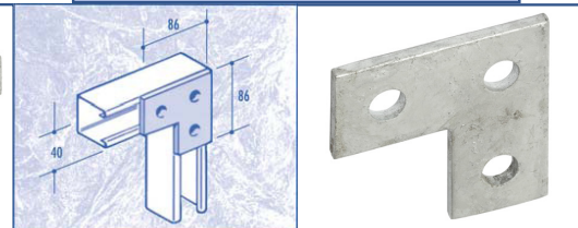
CF6 'L' BRACKET
